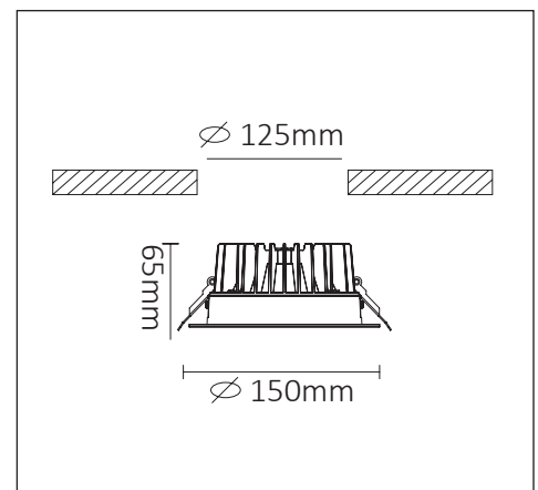
DIMENSIONS
